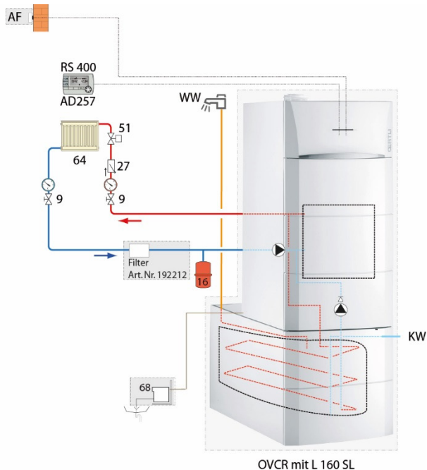
OVCR mit L 160 SL
