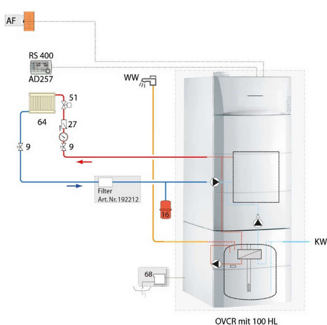
OVCR mit 100 HL
